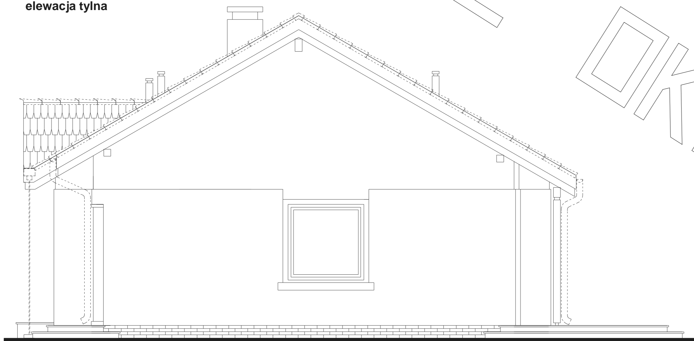
elewacja boczna
