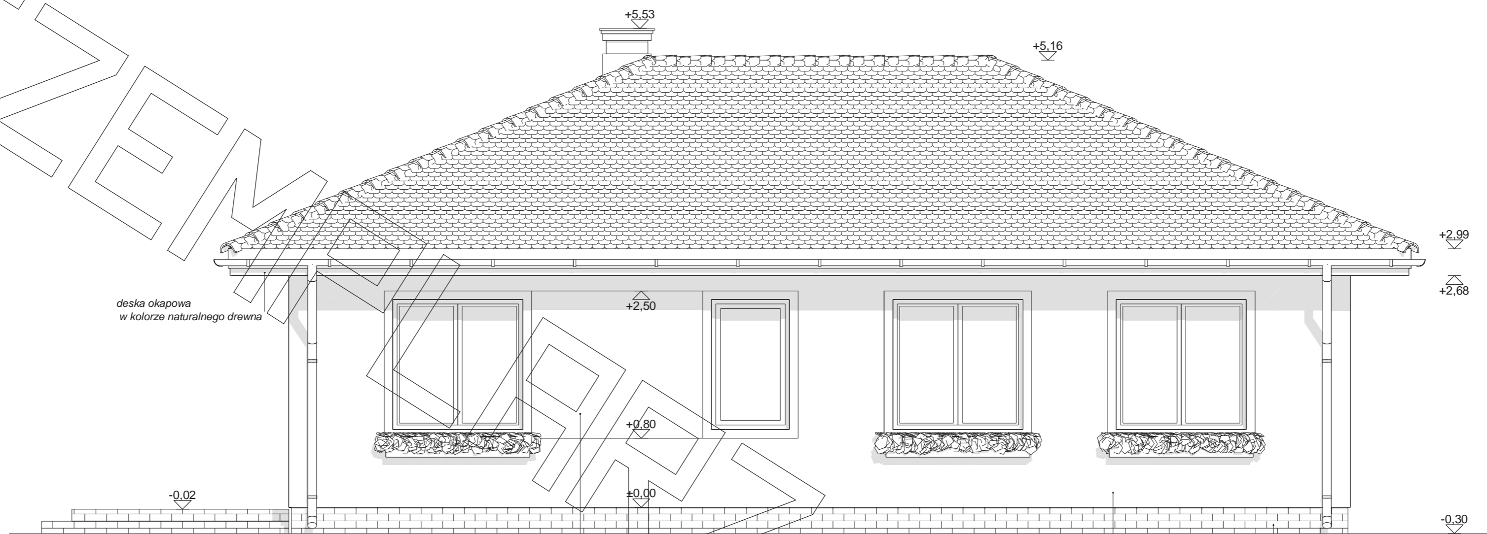
Elwacja tylna
