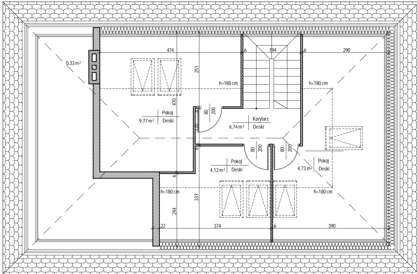
RZUT PODDASZA
