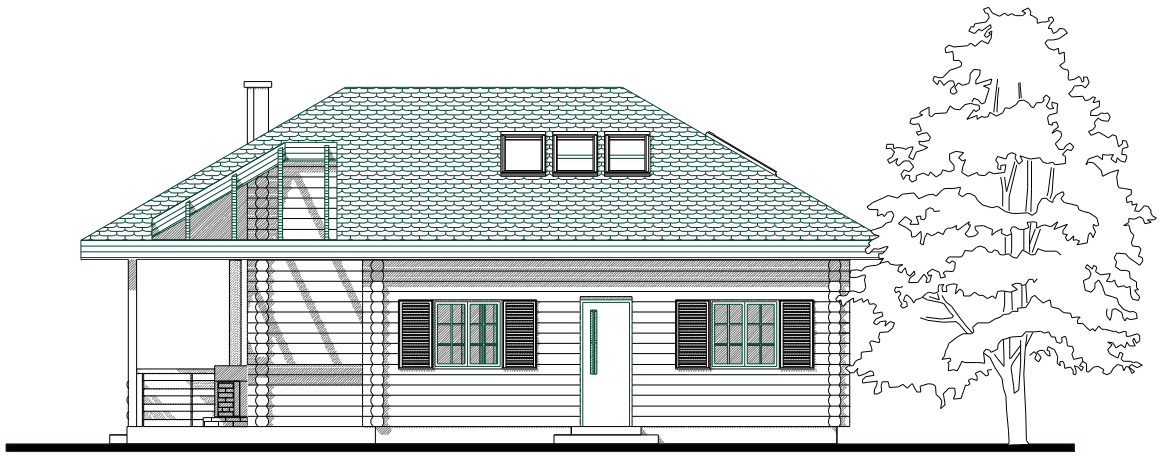
ELEWACJA FRONTOWA
