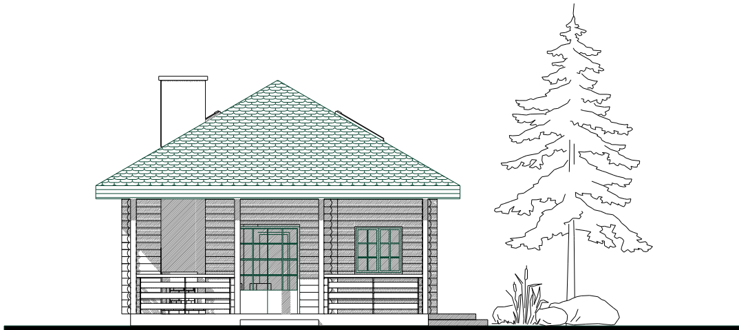
ELEWACJA BOCZNA
