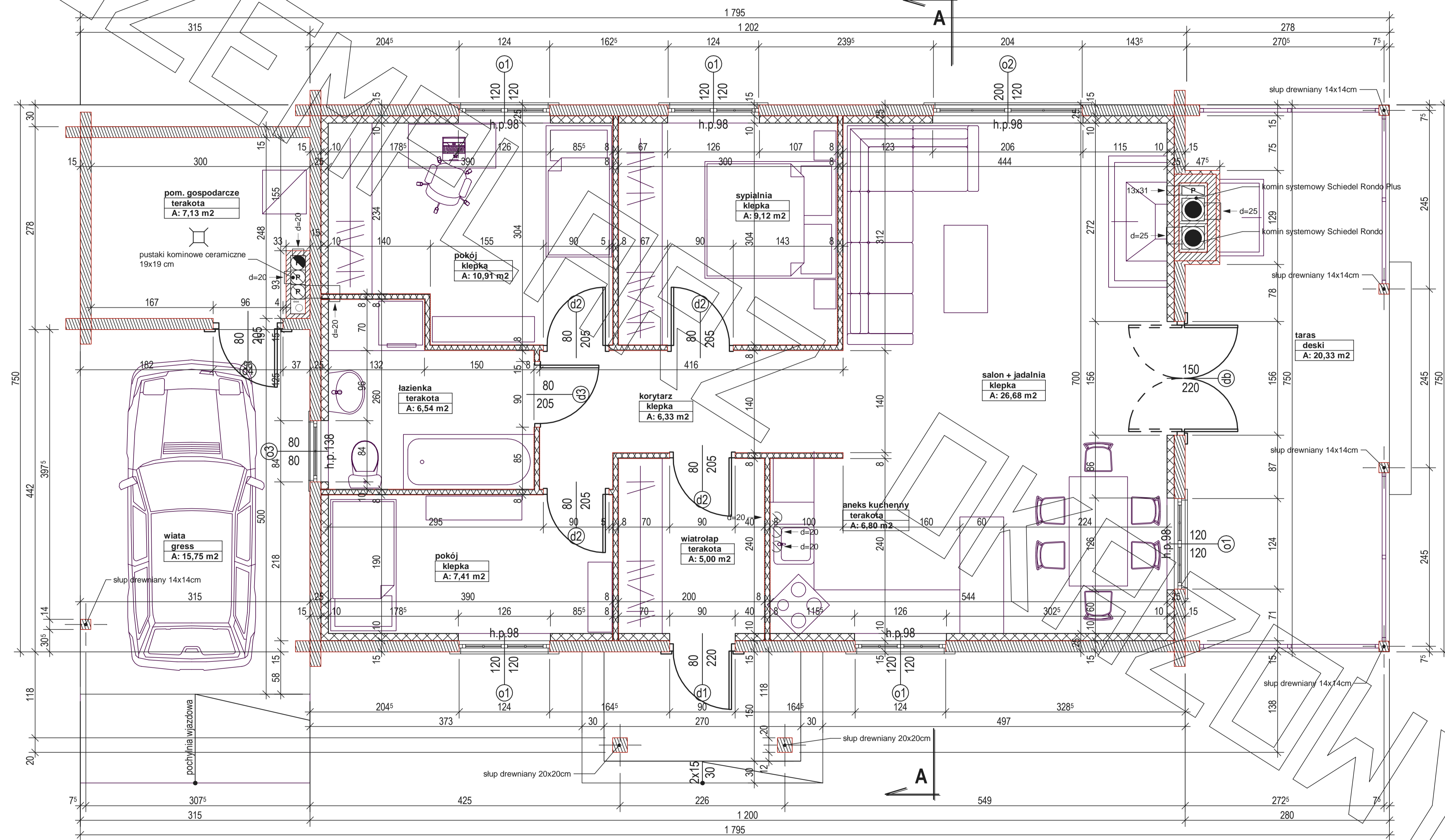
RZUT PARTERU
