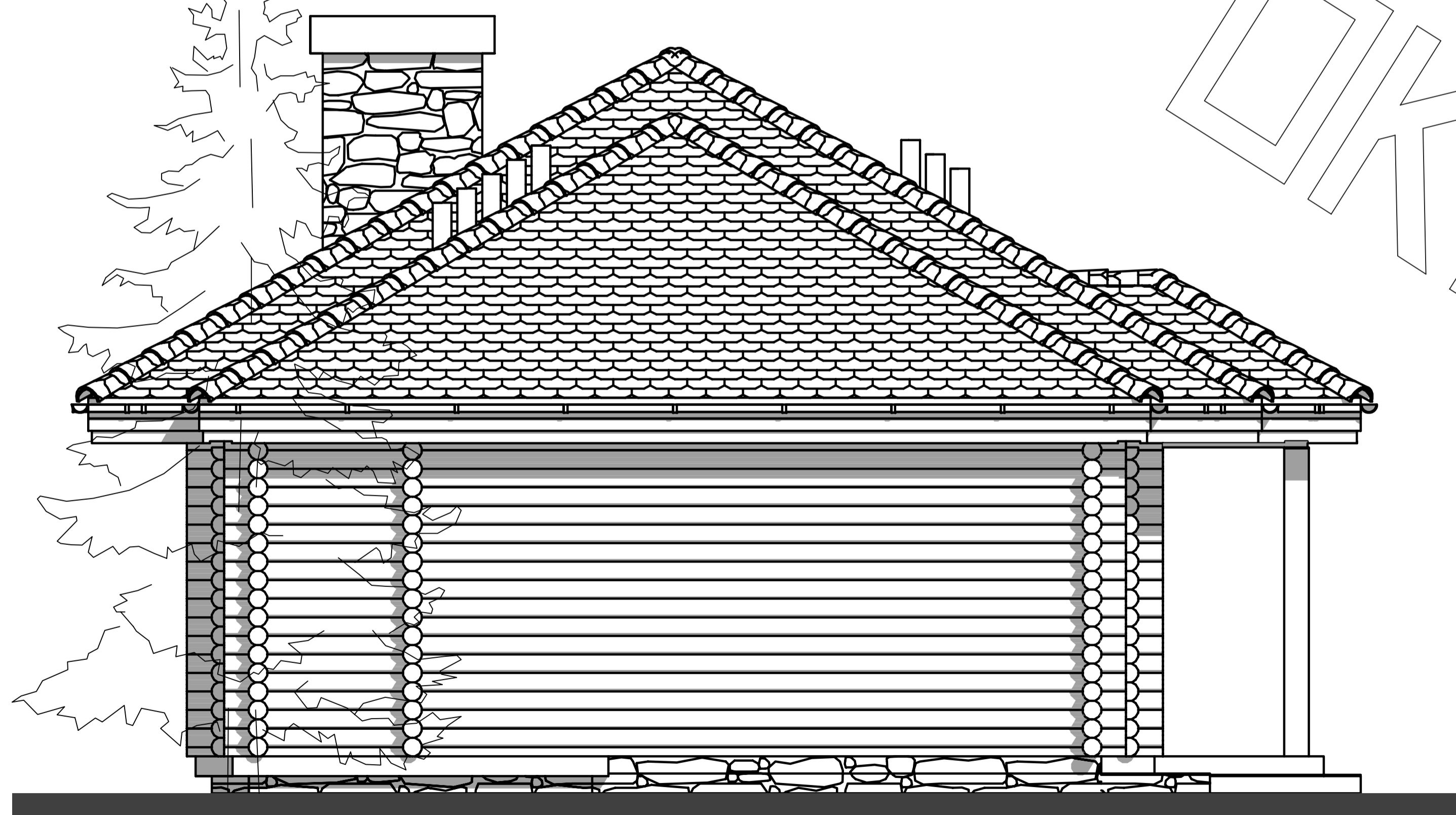
ELEWACJA BOCZNA
