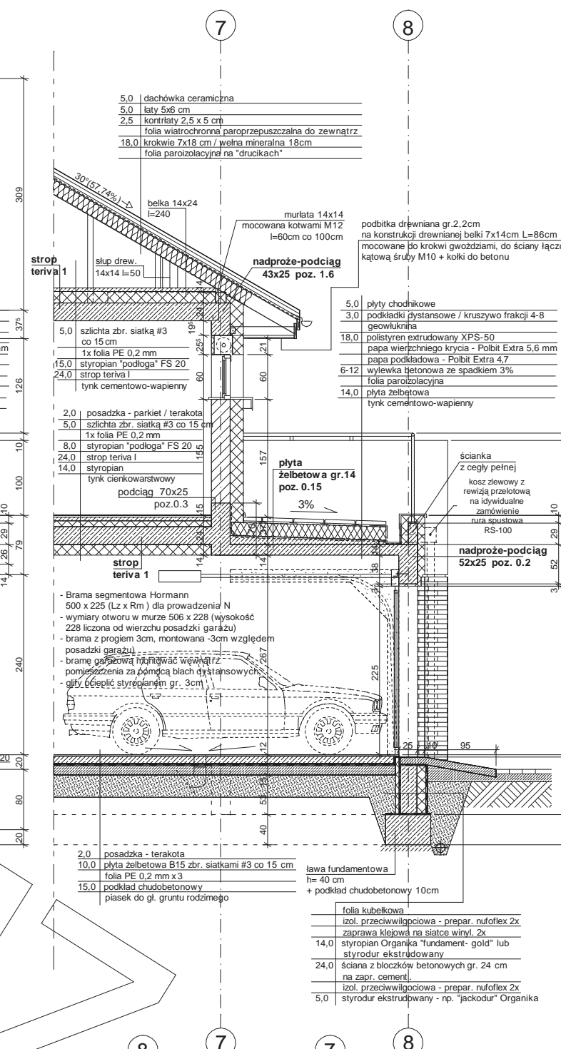
Przekrój B'-B''
