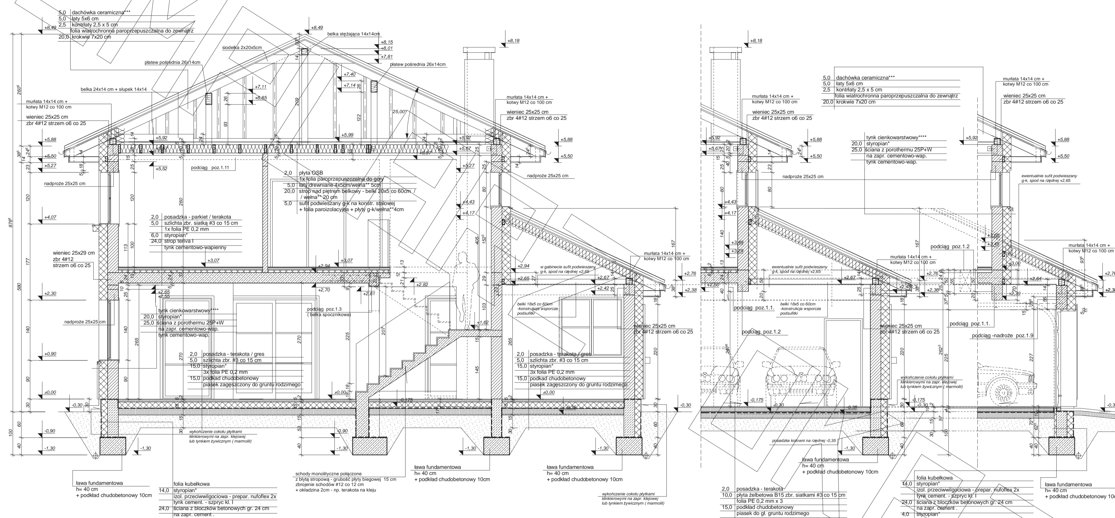
PRZEKRÓJ POPRZECZNY (PRZEZ KLATKĘ SCHODOWĄ) :
