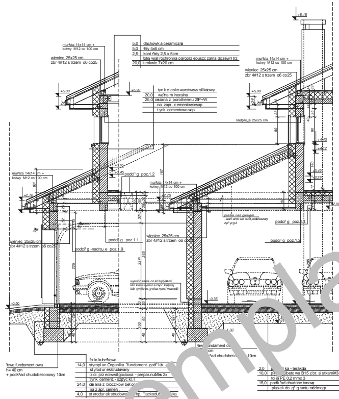
FRAGMENT PRZEKROJU PODDŁUGOWEGO (PRZEZ BRAMĘ GARAŻU):
