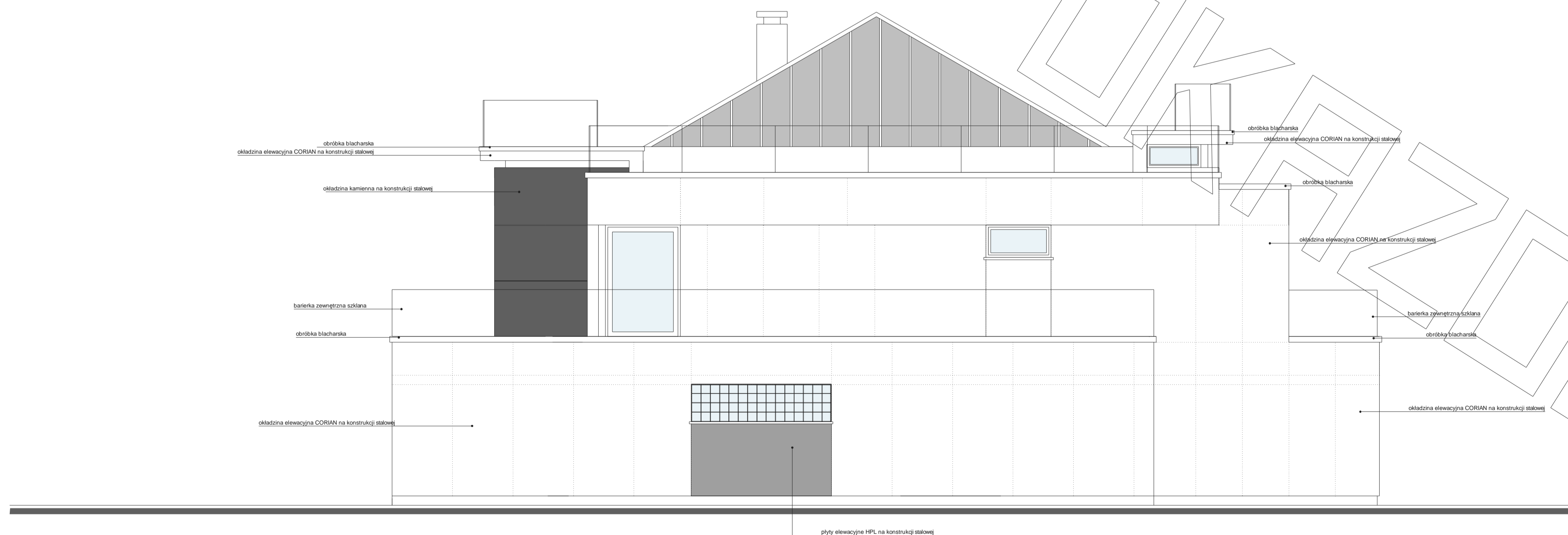
ELEWACJA BOCZNA :
