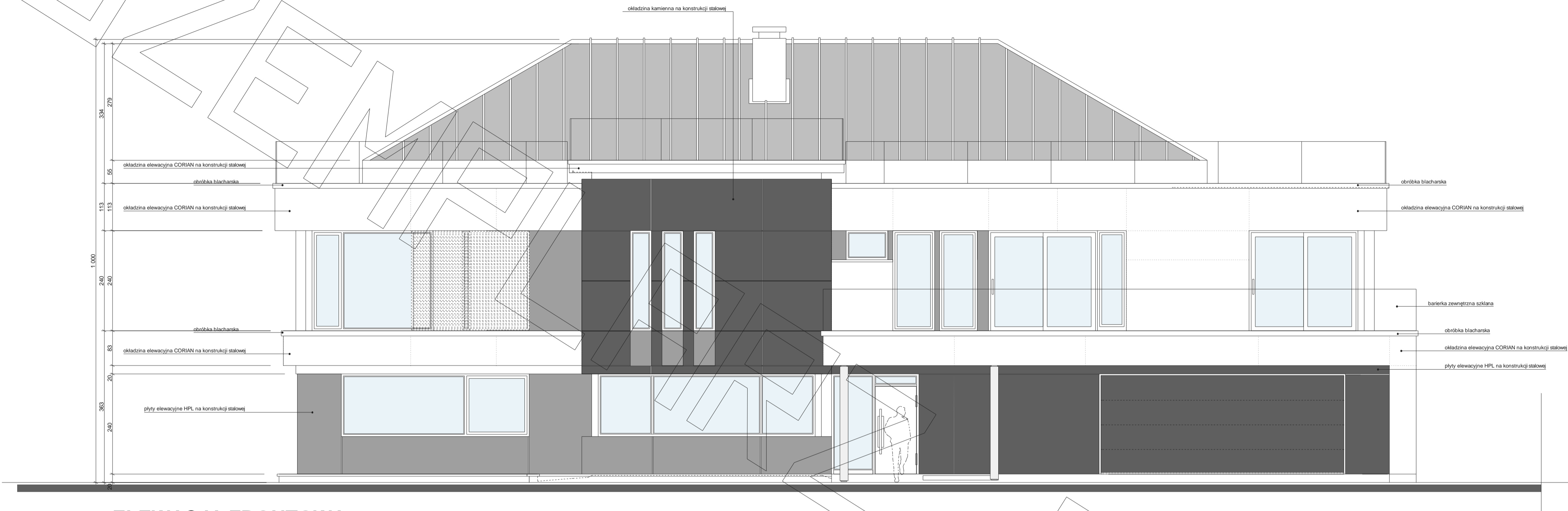
ELEWACJA FRONTOWA :
