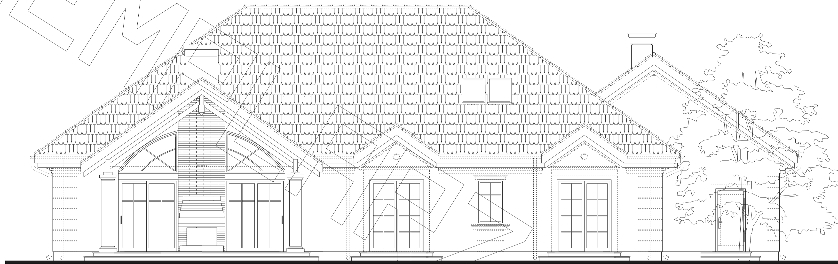
ELEWACJA TYLNA
