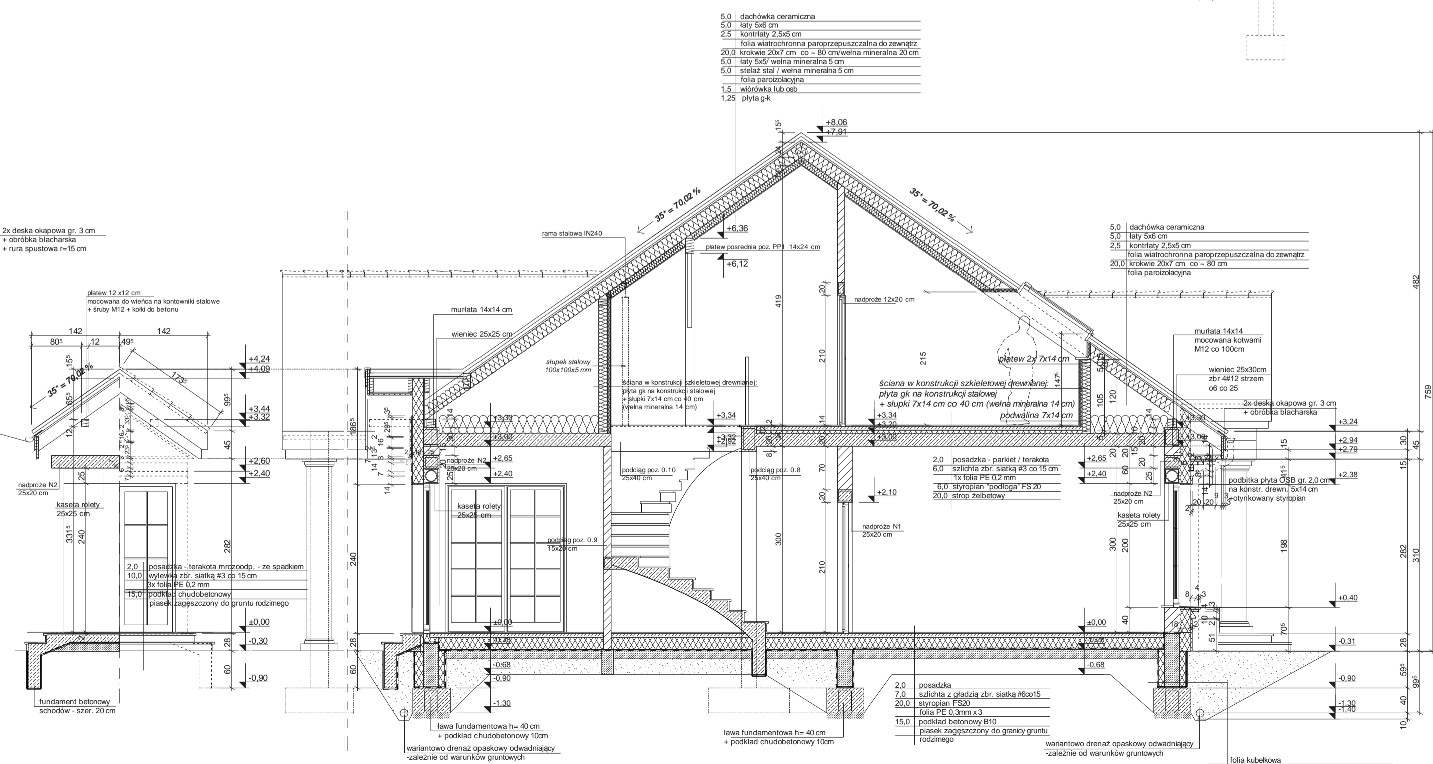
PRZEKRÓJ B-B
